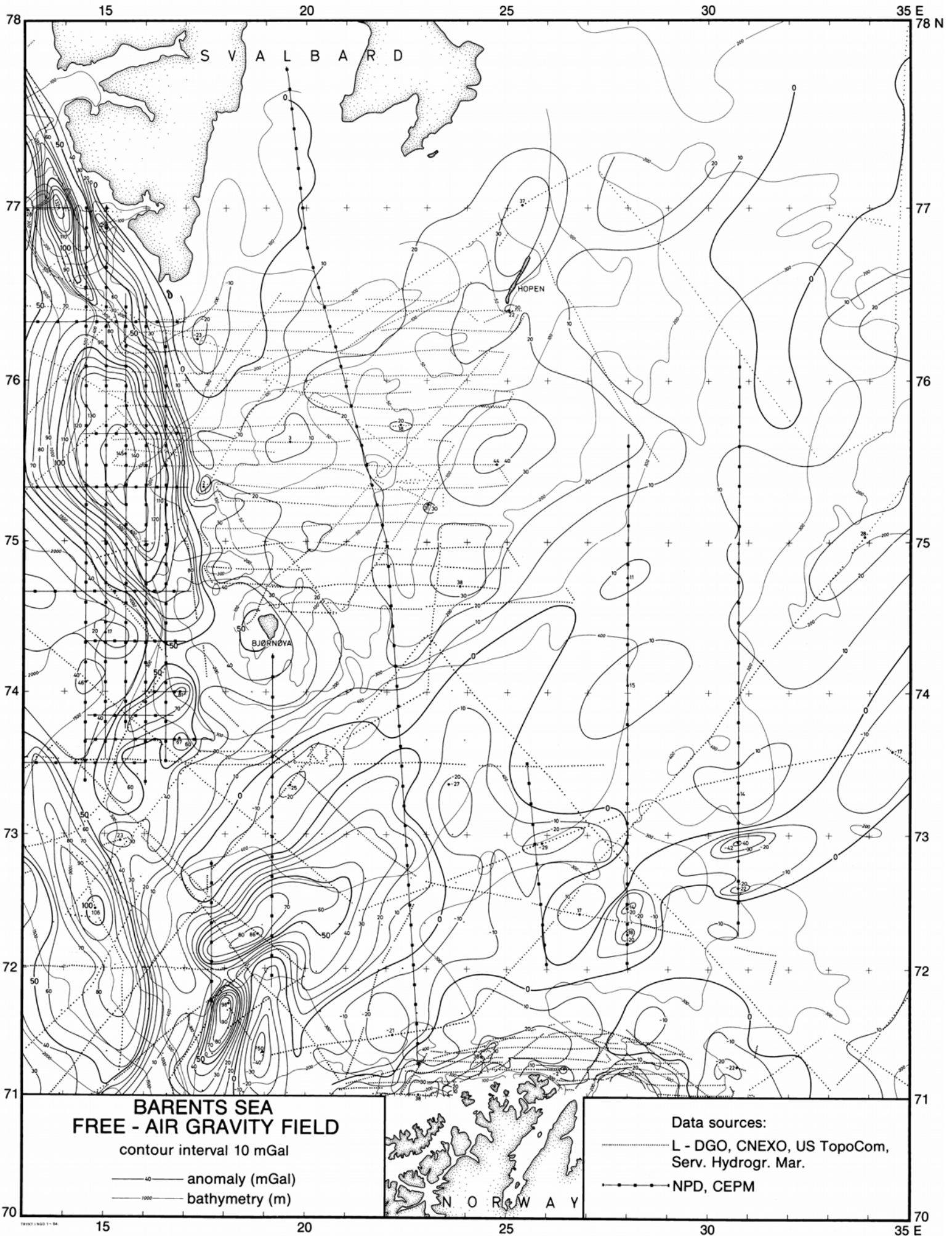
Fig. 3. Free-air gravity anomaly map of the Barents Sea. Bathymetry from Faløide & Godlaugsson (1981). Enclosure Norsk Polarvitenskapelig Skrifte Nr. 180 (1984).
