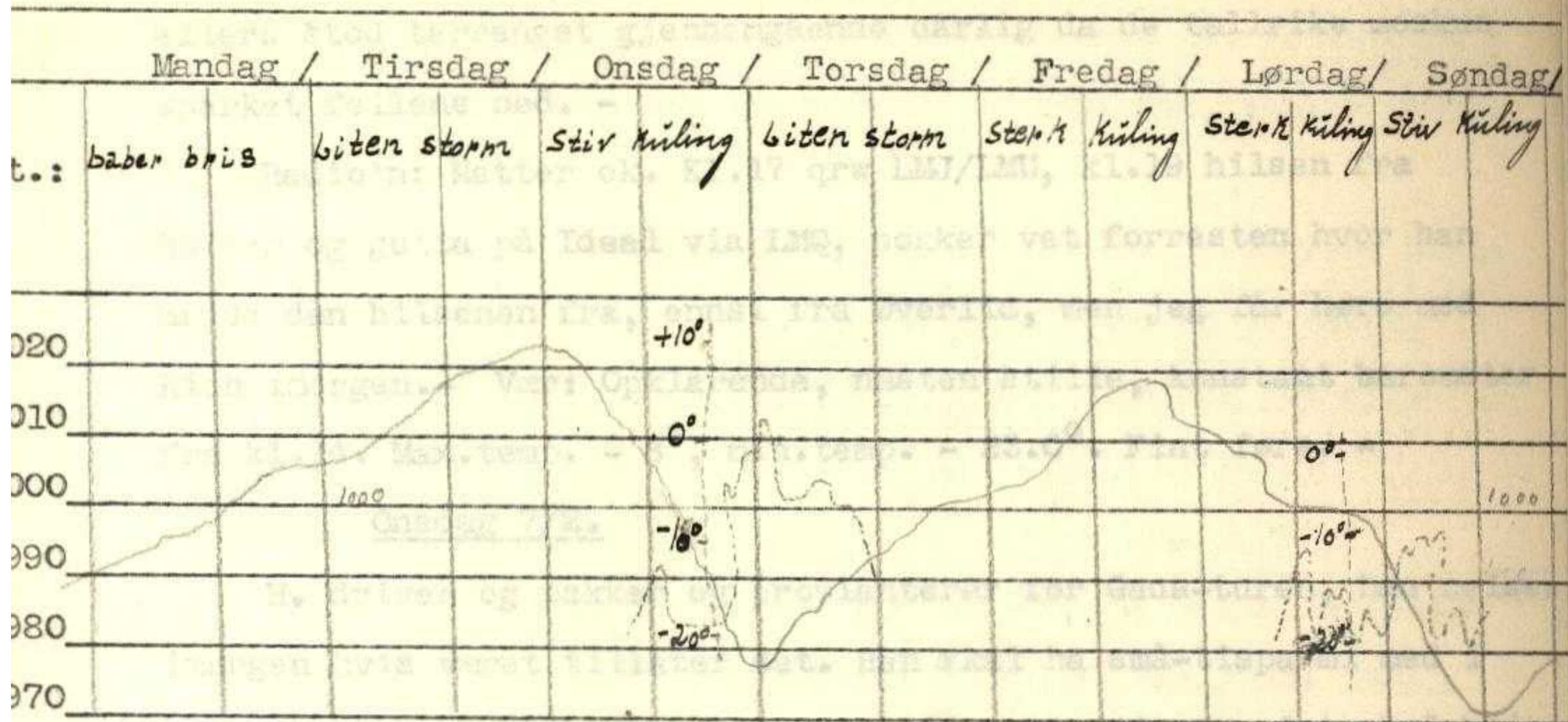
Barogram 29/1 - 5/2 1934. + Temperatursvingninger under stormbyger.
