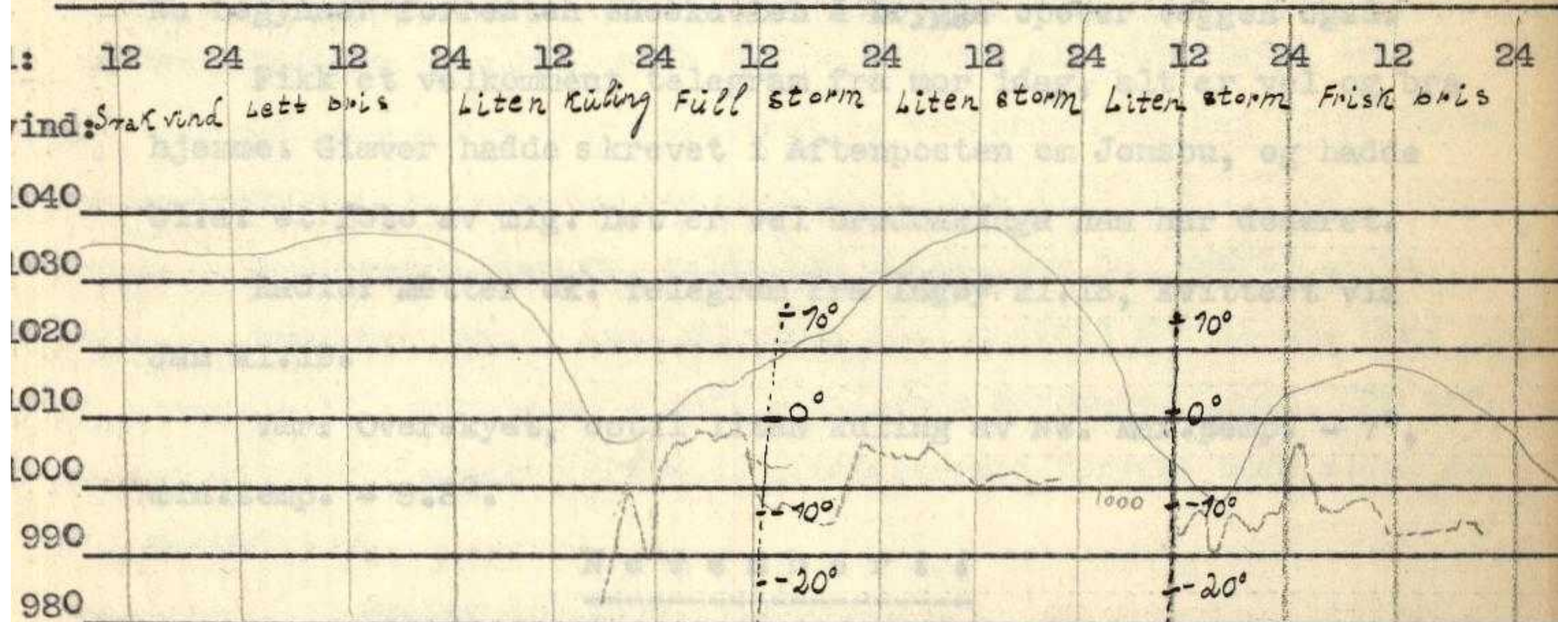
Barogram 23/10 - 30/10 med inntegnet temp. - kurve i storm-perioder.
