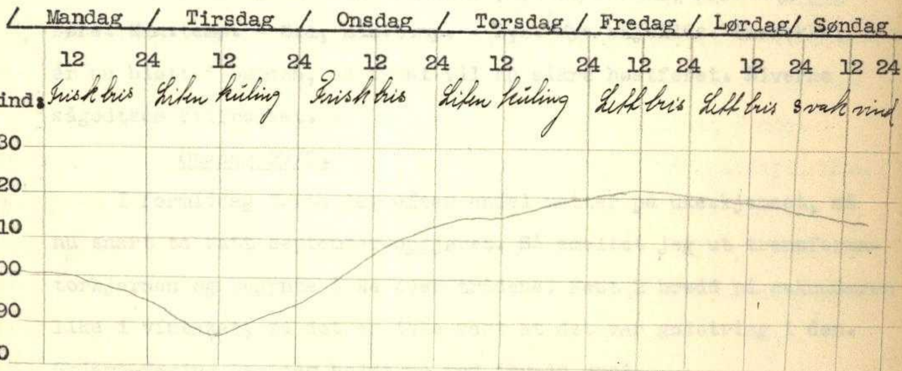
Brøgram 18/9 - 25/9 1933.
